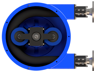
Peristaltic Pumps
